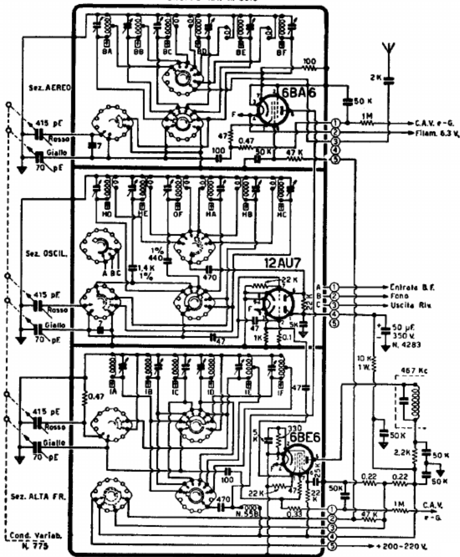
Schema elettrico del Gruppo sintonizzatore N. 2615.
